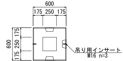
ポール基礎 □600×H500～1500
