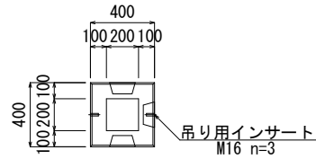
ポール基礎 □400×H500～1500
