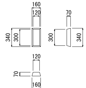
ノックアウト部詳細図
