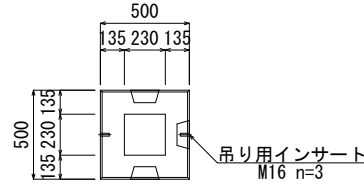
ポール基礎 □500×H500～1500
